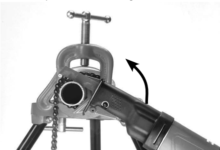
Figura 15A – Cortar o tubo
