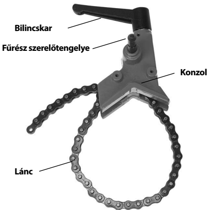
2. ábra – Támasz
