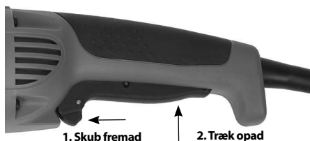
Figur 9 – Kontaktbetjening
