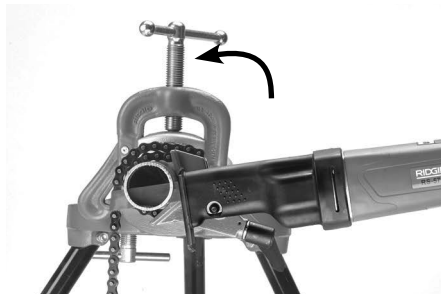
Figuur 15B– De pijp zagen
