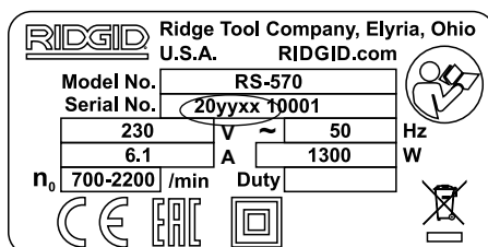
Figur 3 – Serieskylt ("20xx" = tillverkningsår. "xx" = tillverkningsvecka)
