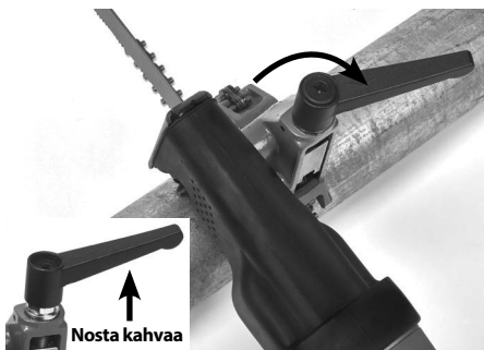
Kuva 14 – Puristuskahvan säätäminen
