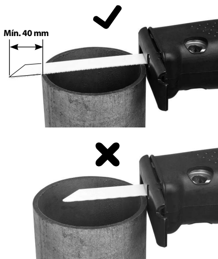
Figura 6 - Longitud adecuada de la hoja
