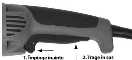
Figura 9 – Operarea întrerupătorului
