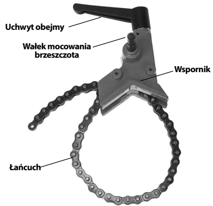
Ilustracja 2 - Urządzenie podporowe
