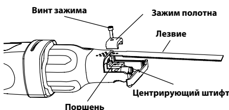
Рис. 7 - Установка полотна
