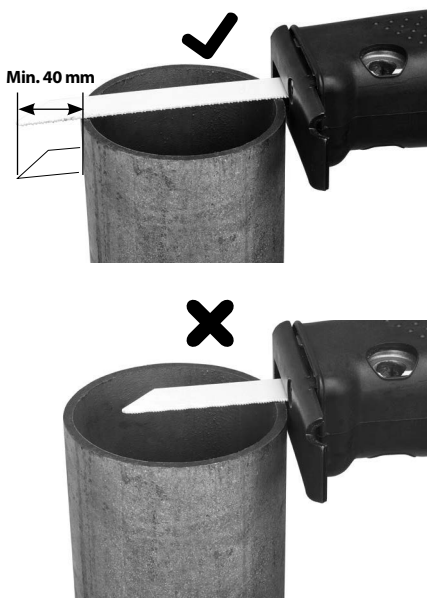
Abbildung 6 – Richtige Blattlänge
