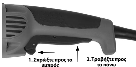
Εικόνα 9 – Λειτουργία διακόπτη
