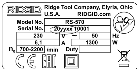
Рис. 3 - Табличка с серийным номером ("20yу" = год производства. "xx" = неделя производства)
