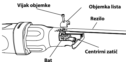
Slika 7 - Nameščanje listov
