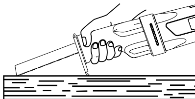
Figur 17A - Dykksskjæring
