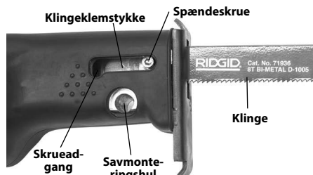
Figur 1 – RS-570 Bajonetsav fra RIDGID®
