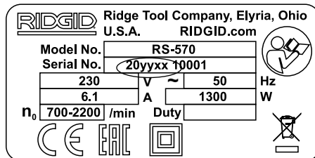
3-сурет – Сериялық тақта («20жж» = Өндірілген жылы. «xx» = Өндірілген аптасы)
