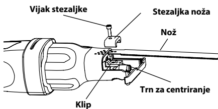
Slika 7 - Ugrađivanje oštrice
