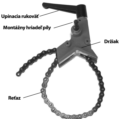
Obrázok 2 – Podporné zariadenie
