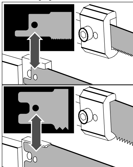
Abbildung 8 – Sitz des Zentrierstifts im Blatt
