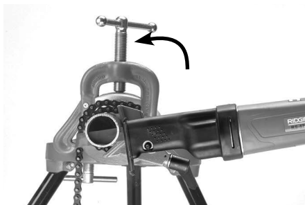
Kuva 15B – Putken leikkaaminen
