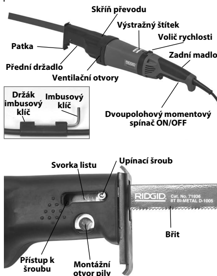
Obrázek 1 – RIDGID® RS-570 přímočará pila
