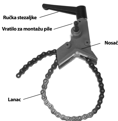
Slika 2 - Uređaj za potporu
