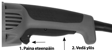
Kuva 9 – Kytkimen toiminta
