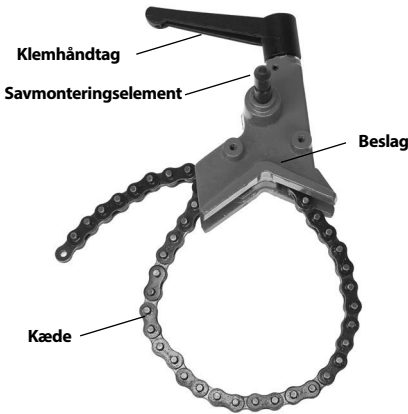
Figur 2 – Støtteanordning (kædeskruestik)
