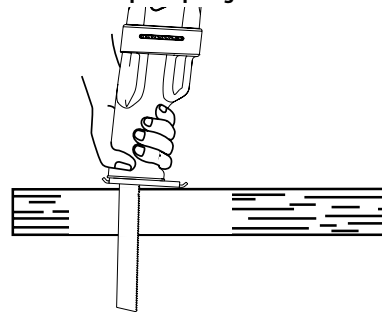
Figure 17C – Découpe en plongée
