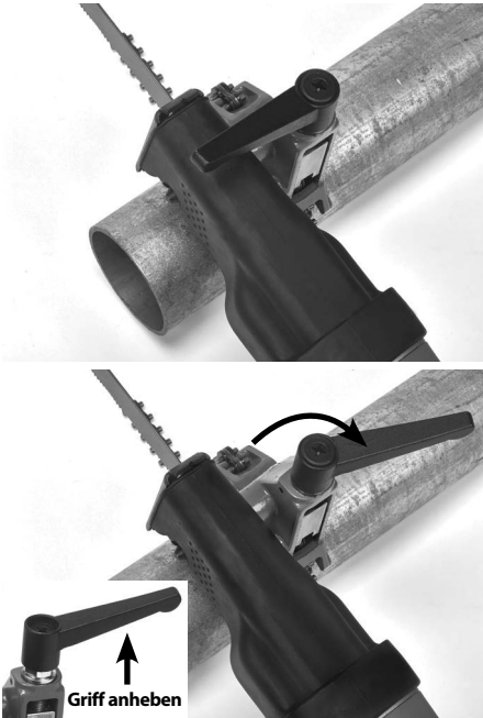
Abbildung 14 – Einstellen des Klemmengriffs
