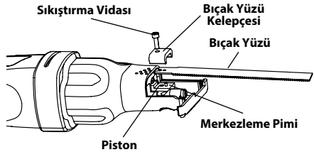
Şekil 7 - Bıçakların Takılması
