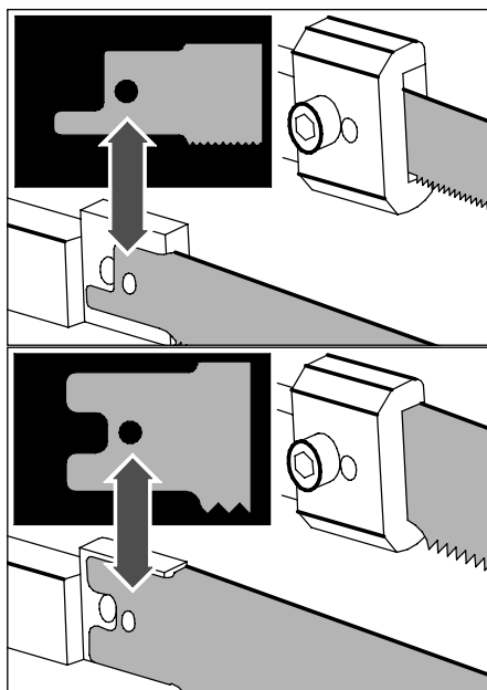
Figura 8 - Acoplamiento del pasador de centrado con la hoja
