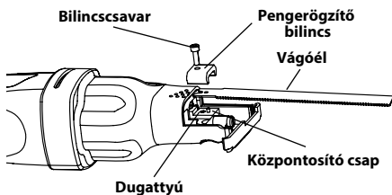
7. ábra – Pengék beszerelése
