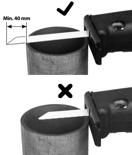
Figur 6 – Korrekt bladlängd
