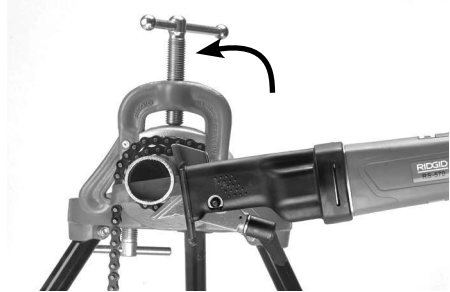
Figura 15B- Corte del tubo
