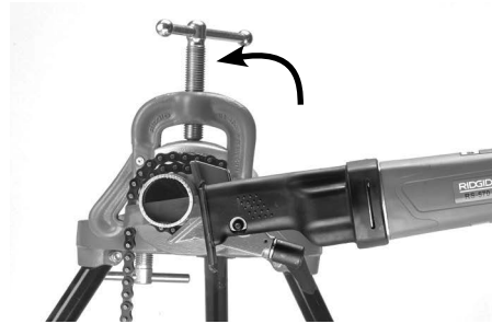
Ilustracja 15B– Cięcie rury
