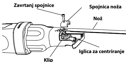
Slika 7 – Postavljanje noža
