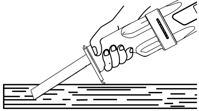
Şekil 17B - Batırma Tipi Kesim
