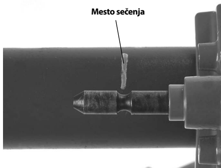
Slika 12 – Postavljanje uređaja za oslanjanje tako da se poravna sa željenim mestom sečenja
