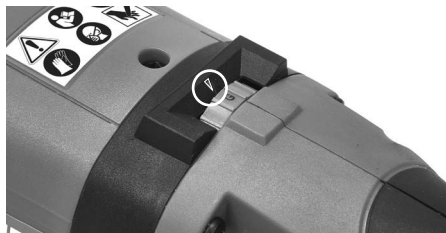
Slika 10 – Nastavitev hitrosti
