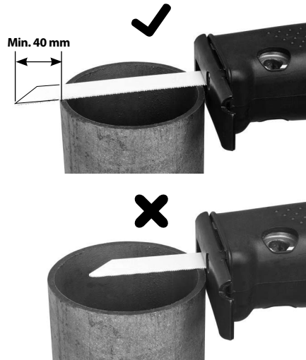
Figur 6 – Korrekt klingelængde
