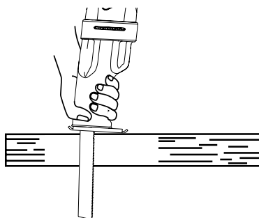
Slika 17C - Potopno žaganje
