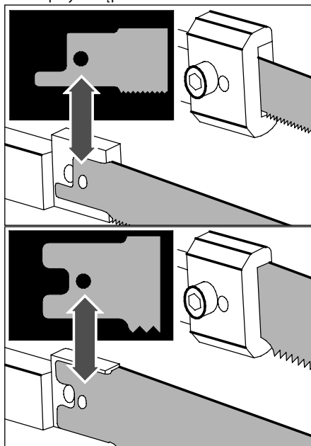
Ilustracja 8 – Zaczepienie trzpienia centrującego w ostrze
