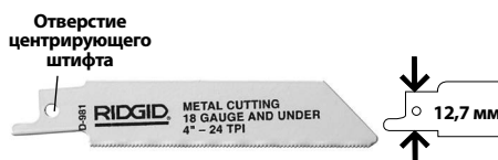
Рис. 5А - Полотна для пил с одинарным хвостовиком
