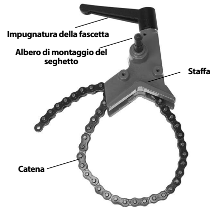
Figura 2 – Dispositivo di supporto
