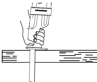
Slika 17C - Rezanje probijanjem
