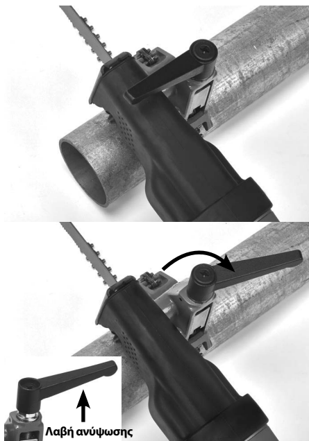
Εικόνα 14 – Ρύθμιση λαβής σφιγκτήρα
