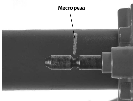
Рис. 12 - Расположение фиксатора для совмещения с требуемым местом реза
