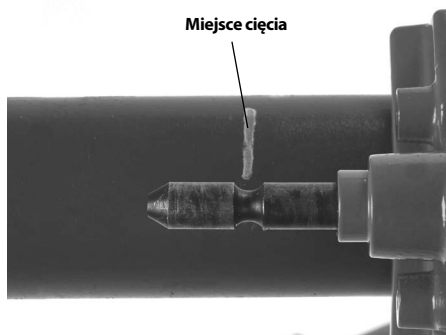
Ilustracja 12 – Umiejscowienie urządzenia podpierającego z ustawieniem względem miejsca cięcia
