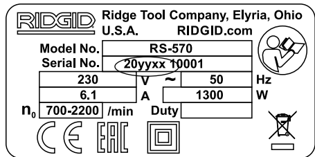
Figur 3 – Plade med serienummer ("20åå" = produktionsår, "xx" = produktionsuge)
