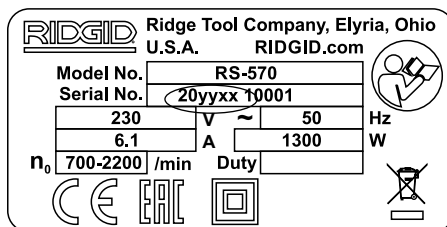
Figur 3 – Serieplate ("20yy" = produksjonsår. "xx" = produksjonsuke)
