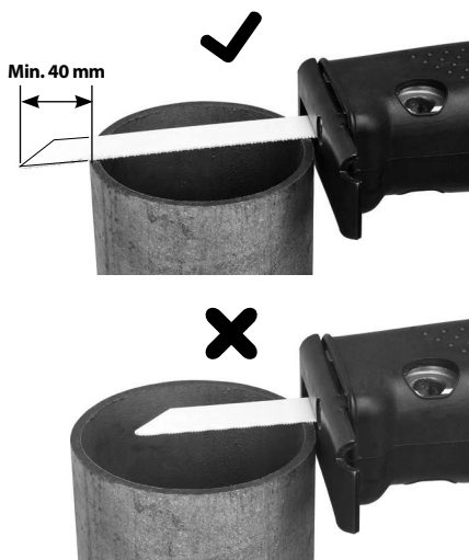
Figuur 6 – Juiste zaagbladlengte
