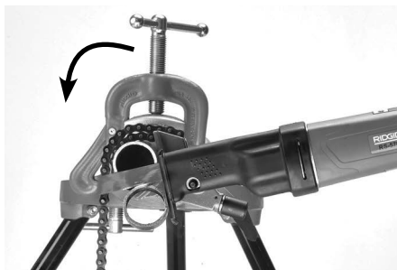
Kuva 15C – Putken leikkaaminen
