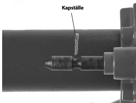
Figur 12 – Stödanordningen ska placeras i linje med det önskade kapstället
