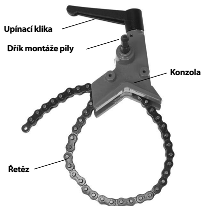
Obrázek 2 – Podpěrné zařízení
