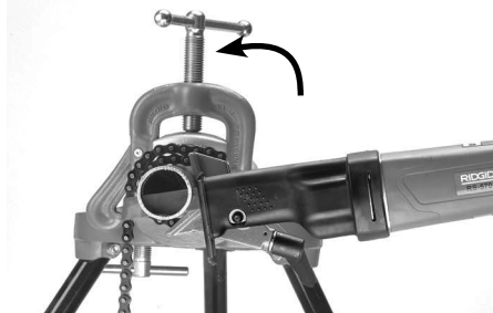
15В-сурет– Құбырды кесу
