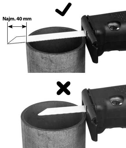
Slika 6 - Pravilna dolžina lista
