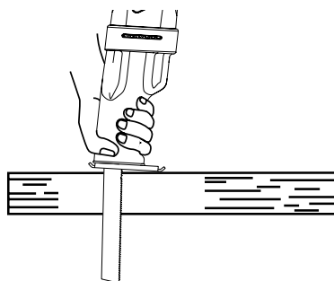
Slika 17C – Ubodno sečenje
