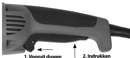
Figuur 9 – Bediening van de schakelaar
