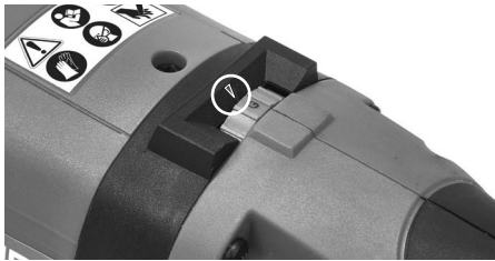
Figura 10 – Reglarea vitezei
