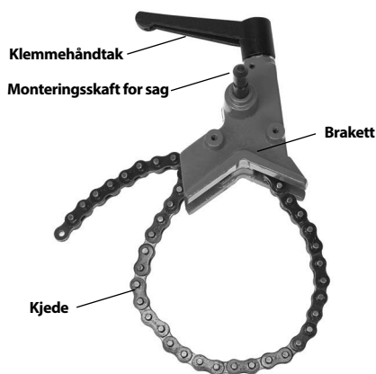
Figur 2 – Støtteenhet
