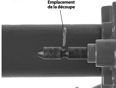
Figure 12 – Positionnement du dispositif de support avec alignement sur l'emplacement de la découpe souhaitée
