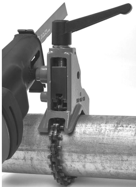
Figur 13 – Montera sågen på stödanordningen
