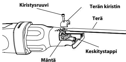
Kuva 7 – Terien asentaminen
