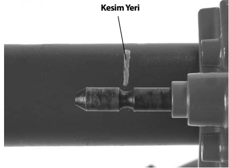
Şekil 12 - Destek Cihazının İstenen Kesik Yeriyle Hizalanacak Şekilde Yerleştirilmesi
