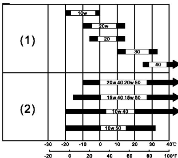
(1)- летние сорта масла, (2)- всесезонные сорта масла
