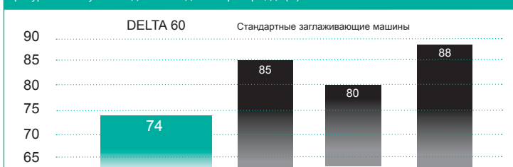
Лр - уровень звукового давления для оператора, дБ(А)
