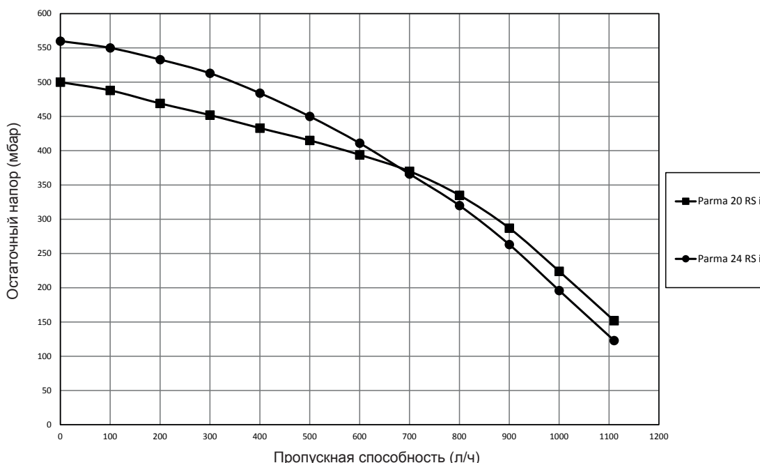
Остаточный напор циркуляционного насоса
