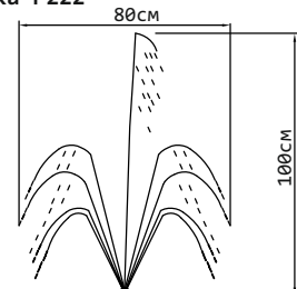
насадка-P222
