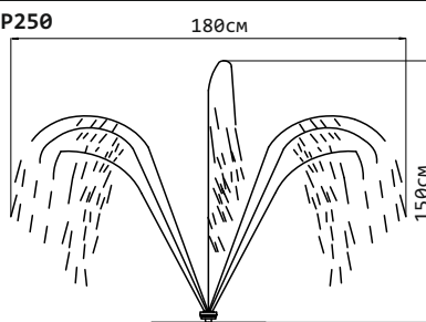
насадка-P250
