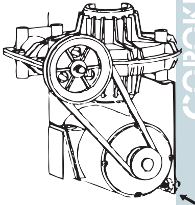
Рисунок 7 – Натяжение клинового ремня электродвигателя стола
