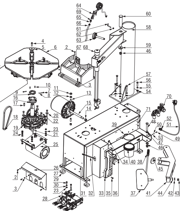
Рисунок 10 – Схема шиномонтажного стенда
