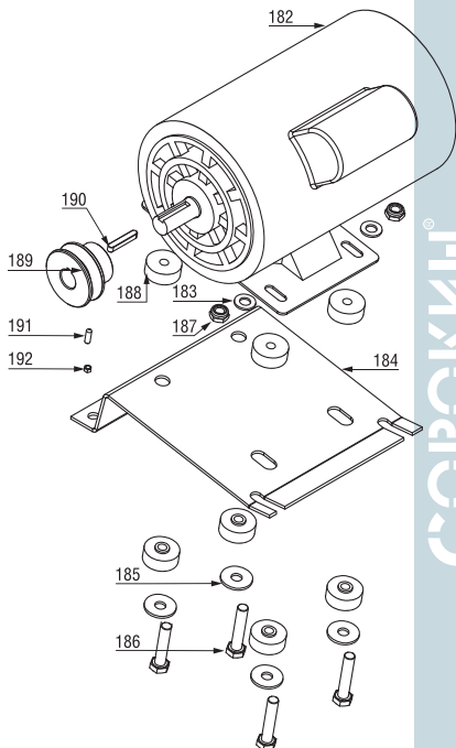
Рисунок 14 – Схема электродвигателя
