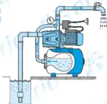
Рис.14 При возобновлении водоразбора, вода, находящаяся в гидроаккумуляторе под давлением, начинает поступать потребителю. Давление в системе при этом постепенно снижается, а насос остается выключенным
