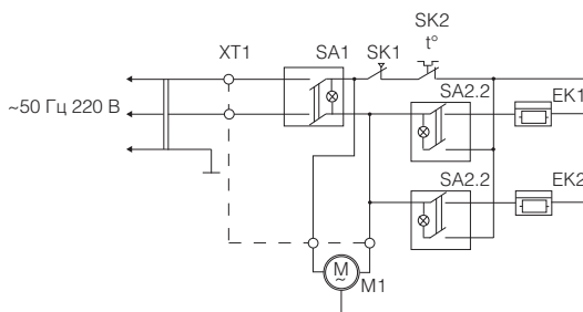
Рис. 1. Схема электрическая тепловентиляторов BHP-3.000
