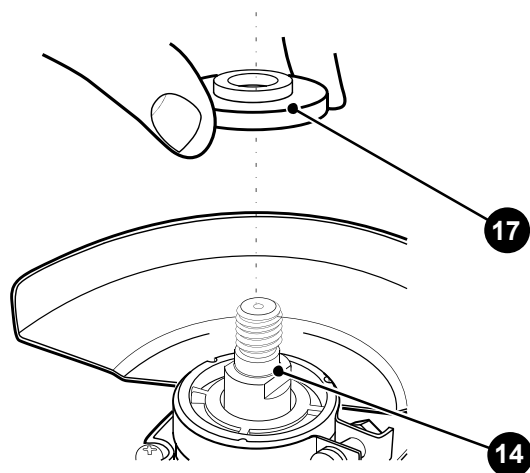
Рисунок С — установка опорного фланца.
