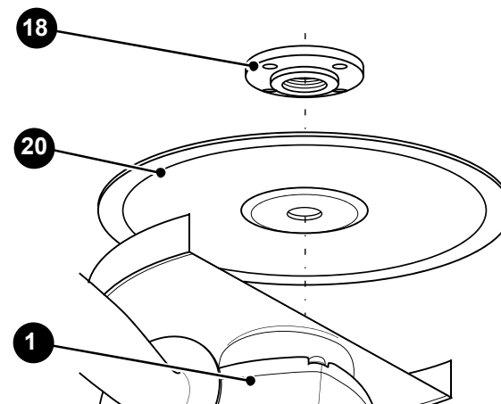
1. Редуктор 18. Зажимной фланец
