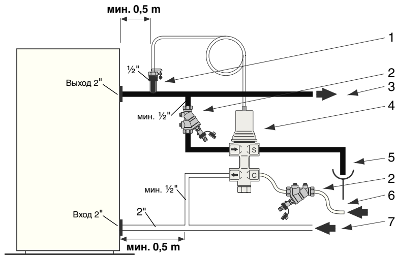
Клапан безопасности Caleffi 544
