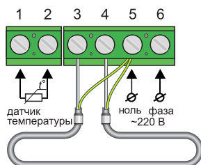
Схема подключения одножильной нагревательной секции ТЛОЭ
