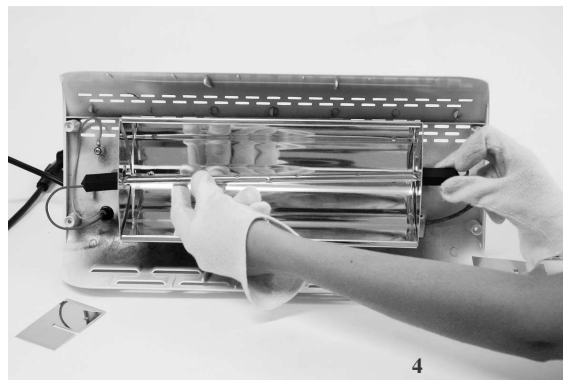
4. ОТСОЕДИНИТЕ ЛАМПУ ОТ УДЕРЖИВАЮЩИХ ЕЕ ЗАЖИМОВ.
