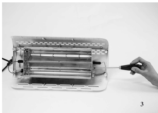
3. ОТКРУТИТЕ ВИНТЫ, ЗАКРЕПЛЯЮЩИЕ НЕБОЛЬШИЕ ЗАЩИТНЫЕ ДЕТАЛИ ПО БОКАМ ОБОРУДОВАНИЯ.
