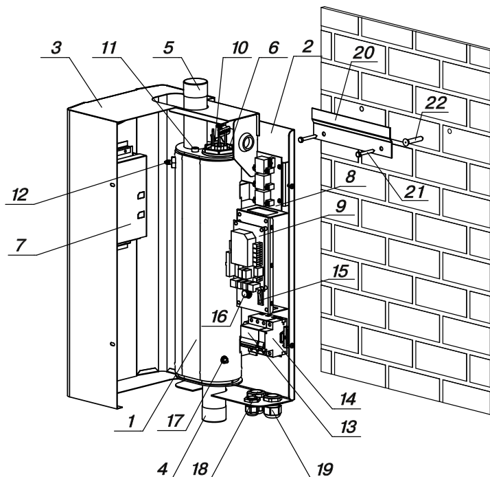
Рис. 1. Конструкция водонагревателя и способ его крепления к стене
