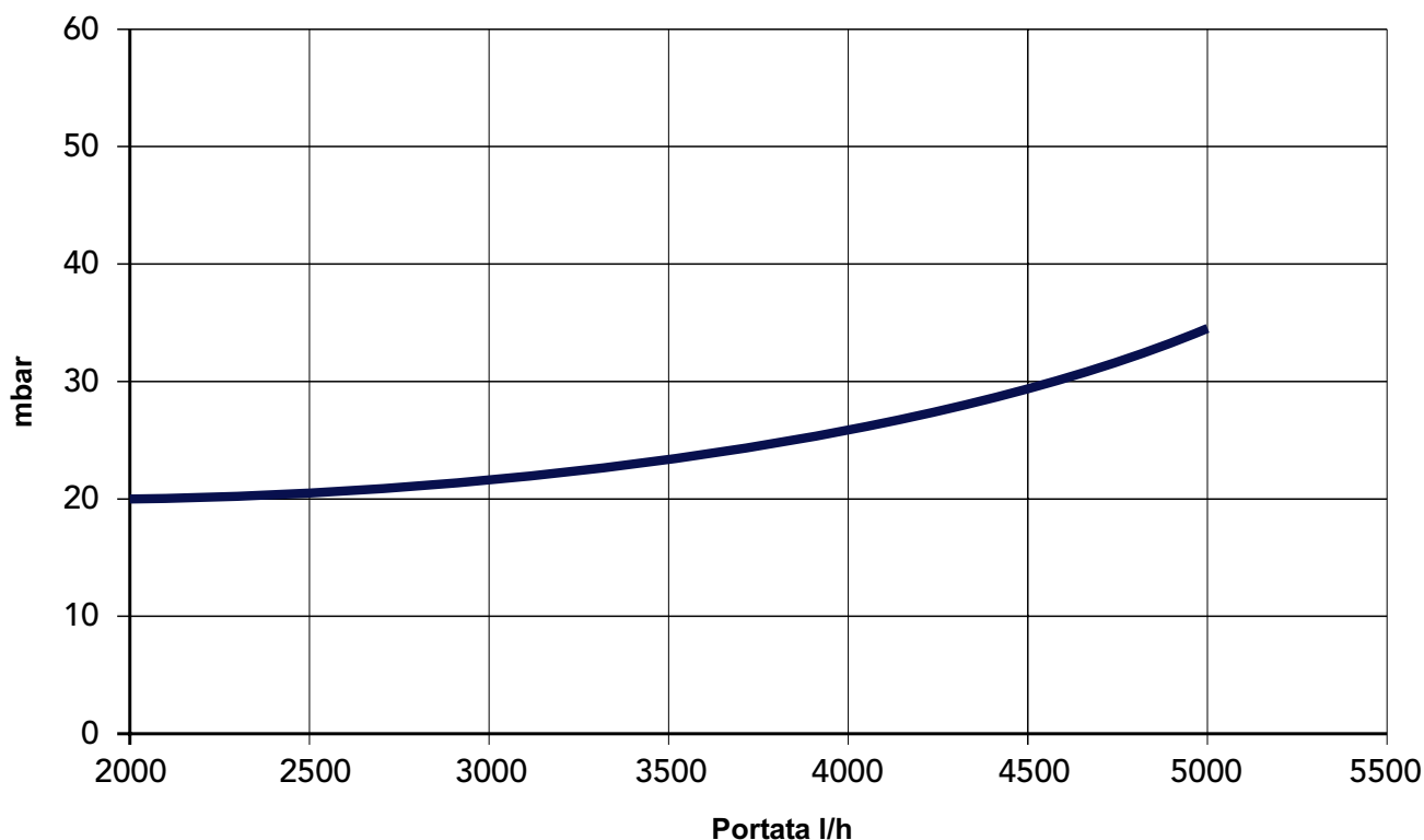
рис. 17 - Соппротивление системы
