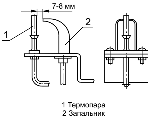
Рисунок 3 - Устройство запальное
