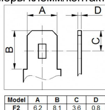
Размеры клемм/контактов F2
