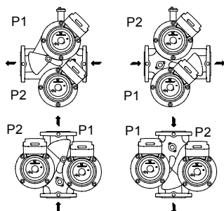
8-сур. Қосарлы сорғыларға арналған ағын бағыты
