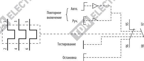
Рисунок 5. Схема электрическая принципиальная реле
