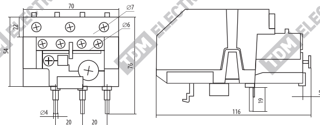
Рисунок 4. Габаритные и установочные размеры реле PTH-3353...PTH-3365, мм
