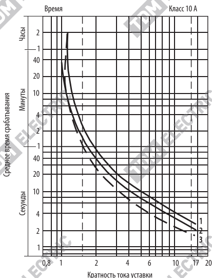
Рисунок 1. Время-токовые характеристики реле
