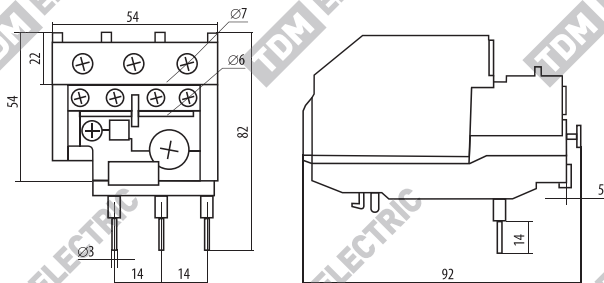
Рисунок 3. Габаритные и установочные размеры реле PTH-2355, мм
