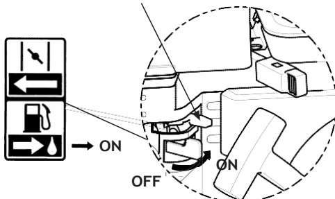
Топливный клапан
