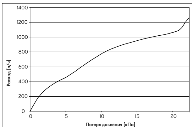
13.1 Потеря давления eIoBLOCK
