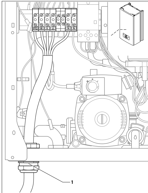
5.1 Подключение к сети (здесь: eloBLOCK VE 24, VE 28)
