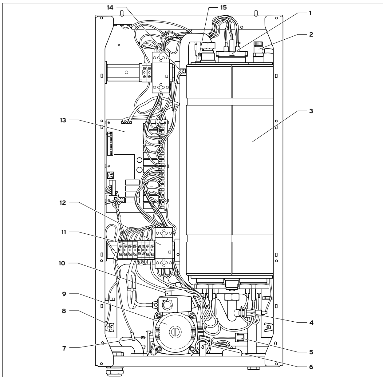
3.1 Вид спереди, аппарат открыт
