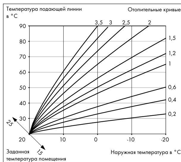
7.1 Настраиваемые кривые отопления
