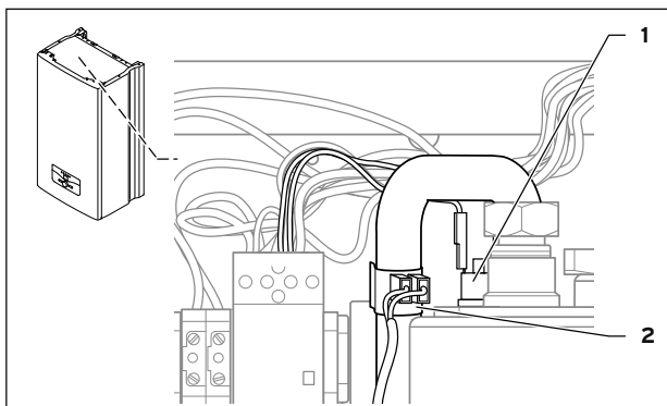
10.9 Датчик температуры NTC и тепловой предохранитель
