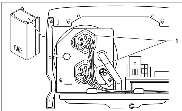
10.6 Демонтаж ТЭНа
