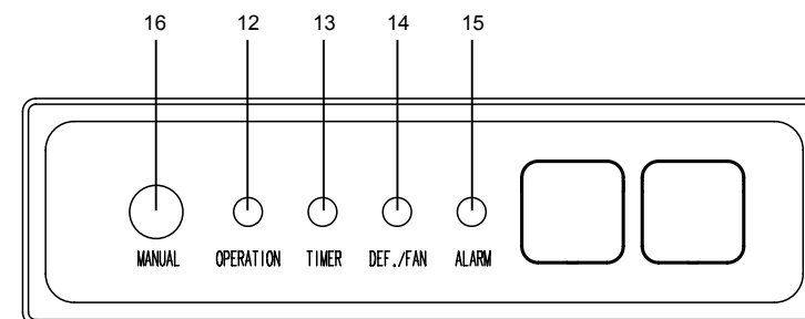
Рис. 2. Описание панели управления внутреннего блока
