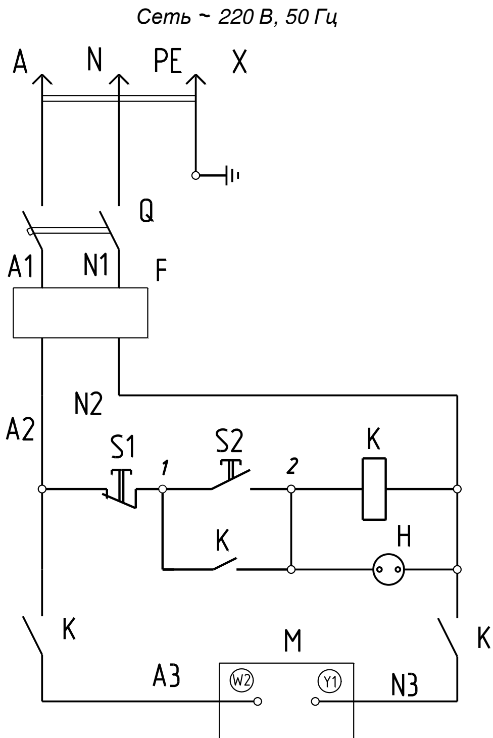
Рисунок 10 - Схема электрическая принципиальная машины СО-206.1 (вариант с однофазным двигателем)
