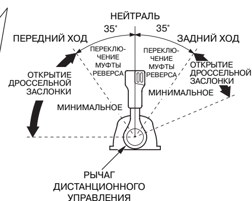
ЗАДНИЙ ХОД
