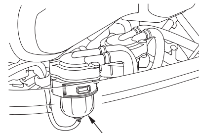
ТОПЛИВНЫЙ ОТСТОЙНИК
