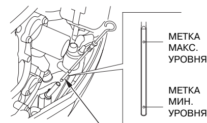
МАСЛЯНЫЙ ЩУП
