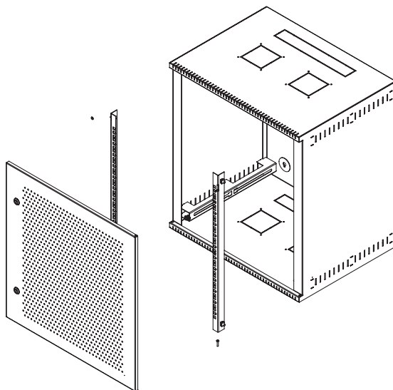
Рис. 1 Разнесенный сборочный чертеж ШТН
